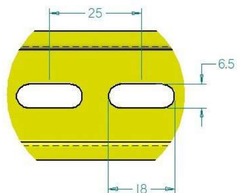
Detalle Oblongos
